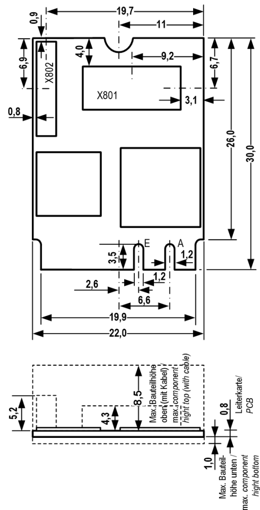
Abbildung 7: Abmessungen CIFX M223090AE (Revision 4)
