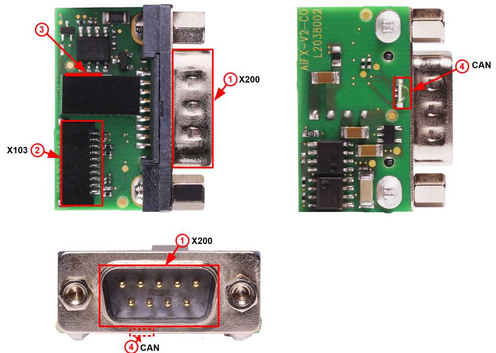
Abbildung 2: Abgesetzte Netzwerkschnittstelle AIFX-V2-CO (Revision 2)
