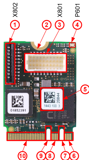
Abbildung 1: Grundkarte CIFX M223090AE (Revision 3)
