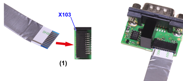
Abbildung 4: Kabel an abgesetzte Netzwerkschnittstelle CANopen AIFX-V2-CO anschließen
