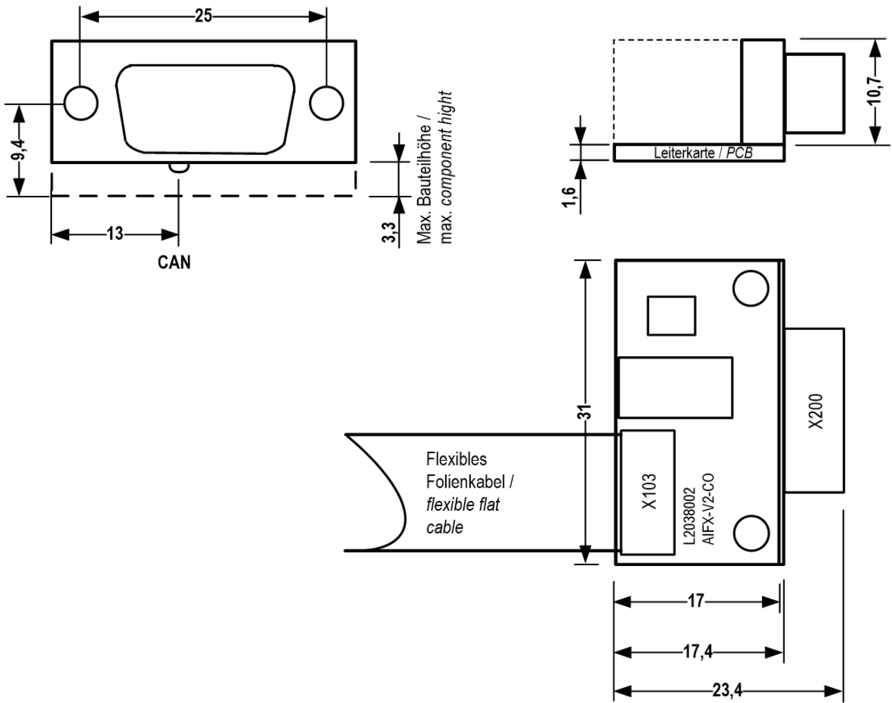
Abbildung 8: AIFX-V2-CO (Revision 3)
