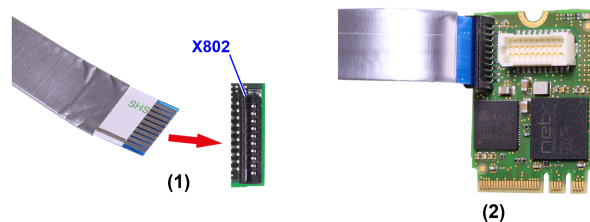
Abbildung 5: Kabel an Grundkarte anschließen, Beispiel CIFX M223090AE
