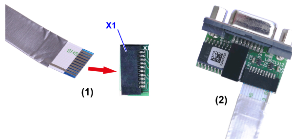
Abbildung 4: Kabel an abgesetzte Netzwerkschnittstelle Feldbus AIFX-DP anschließen
