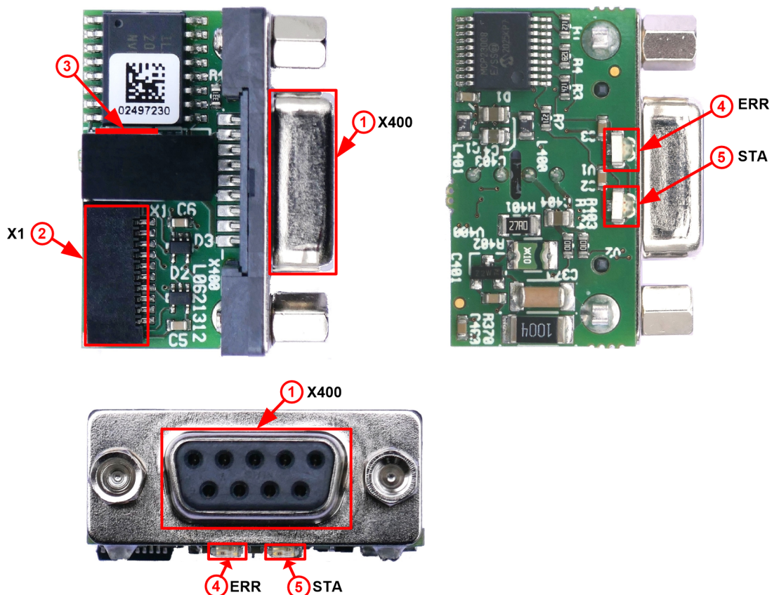
Abbildung 2: Abgesetzte Netzwerkschnittstelle AIFX-DP (Revision 2)
