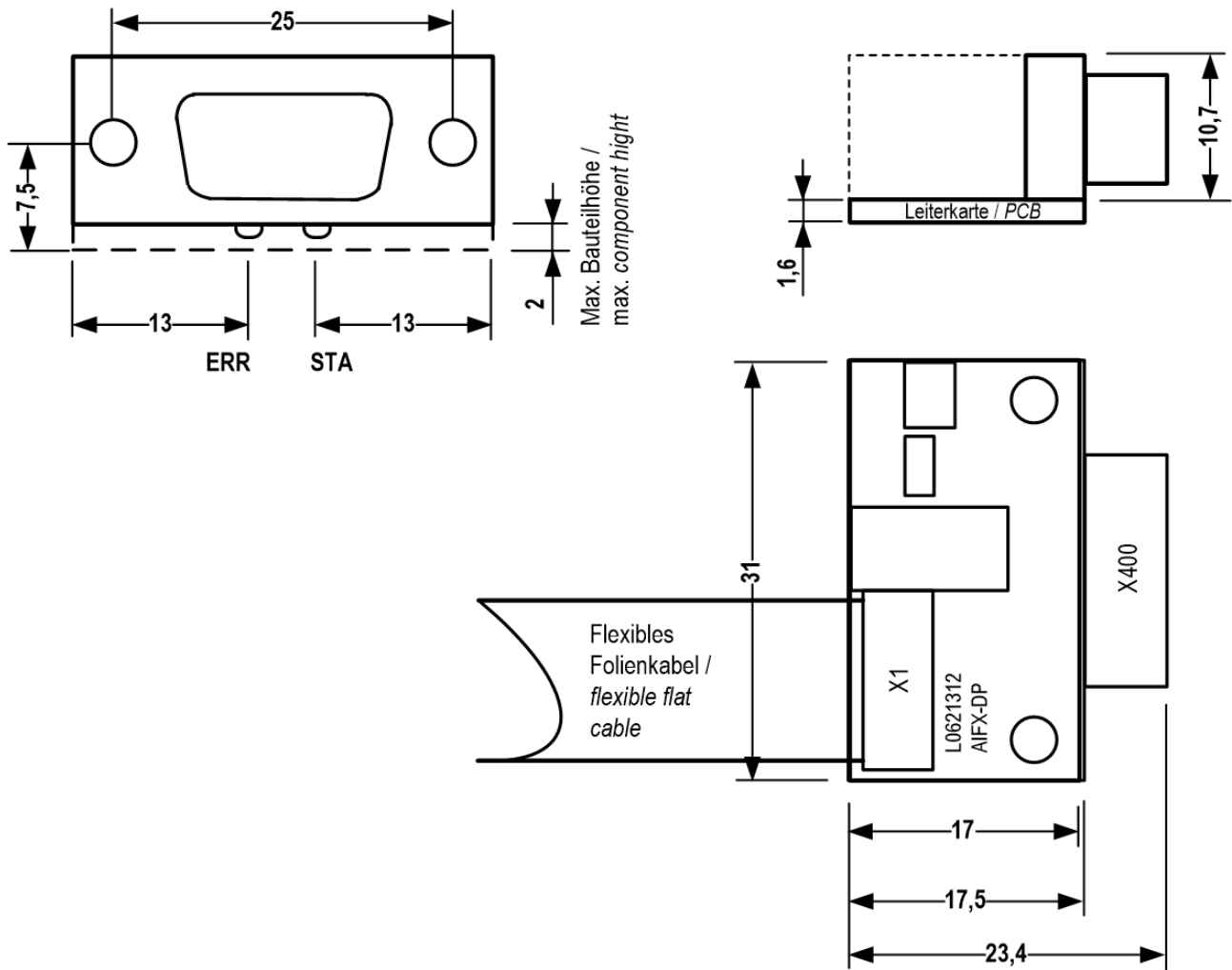
Abbildung 8: AIFX-DP (Revision 2)
