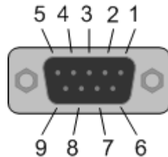
Abbildung 6: PROFIBUS-Schnittstelle (DSub-Buchse, 9-polig), X201
